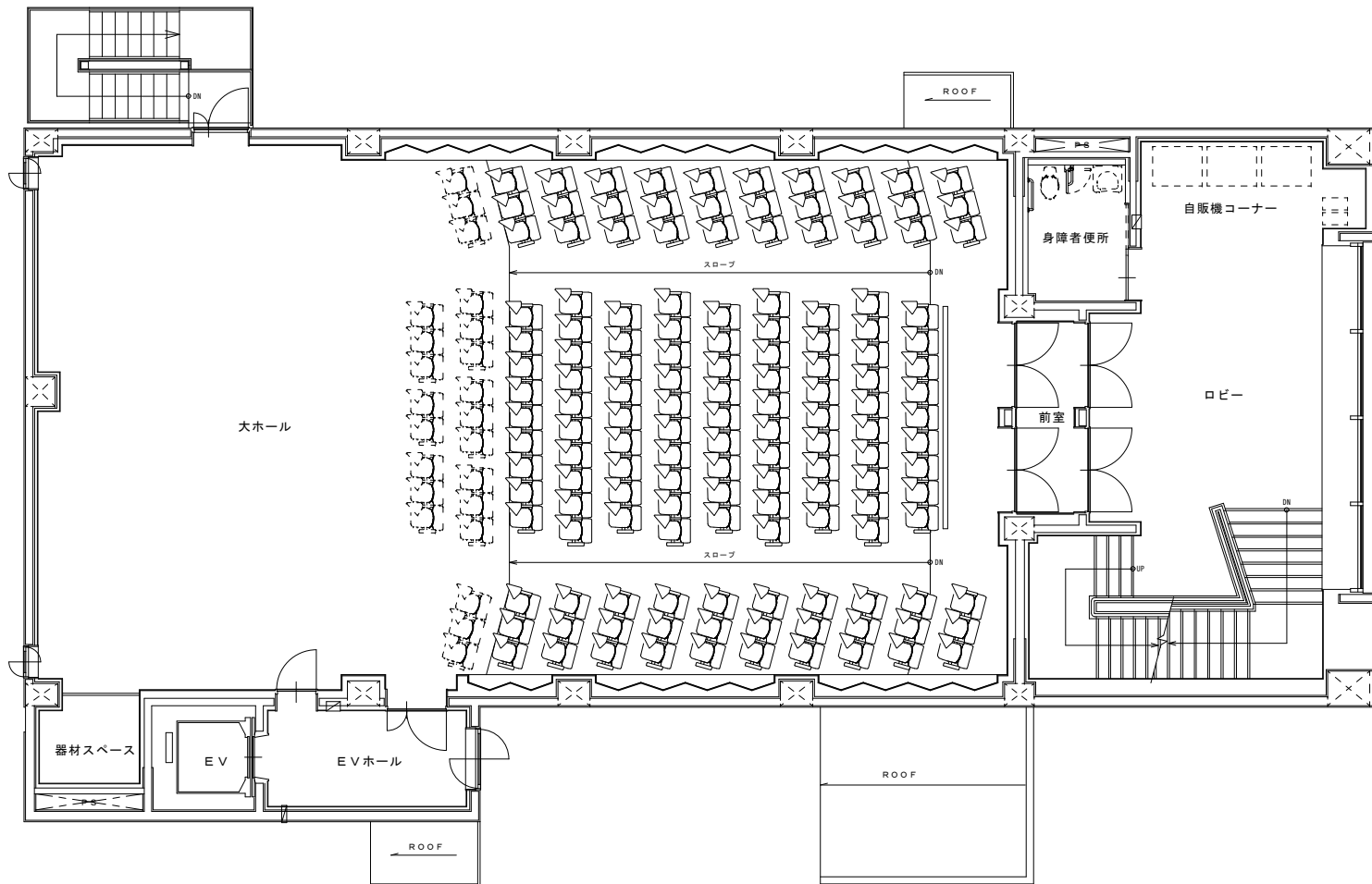
2階平面図
